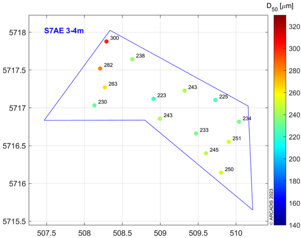
Figuur 6-4 Ruimtelijke variatie in D 50 op een diepte van 2-3 m en 3-4m onder het oppervlak in zandwinvak S7AE.
