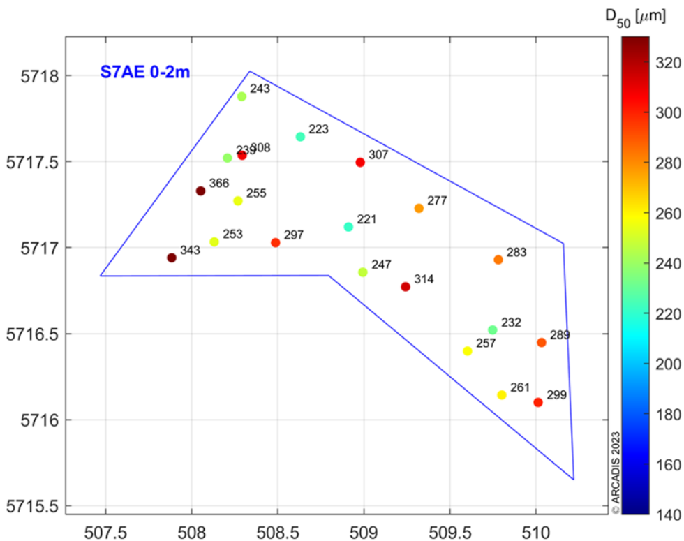
Figuur 6-3 Ruimtelijke variatie in D_{50} op een diepte van 0-2 m onder het oppervlak in zandwinkvak S7AE.
