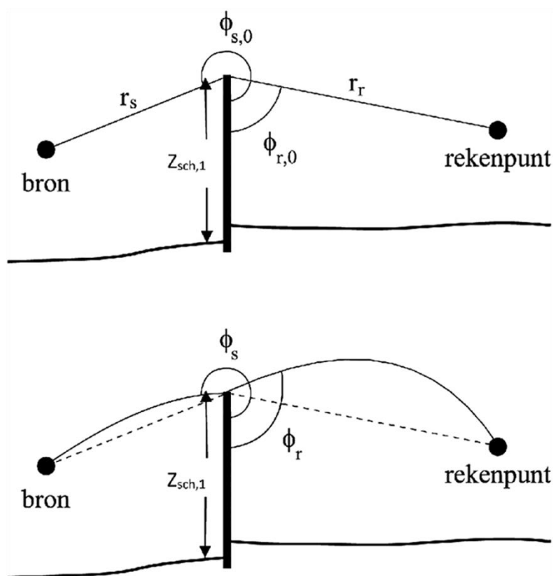
Figuur 4.10: Straalkromming
