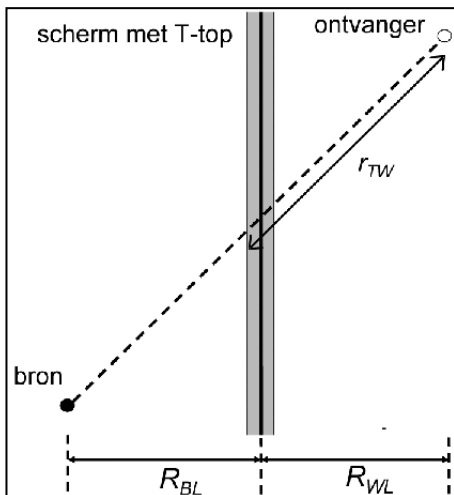
Figuur 5.3 Boveenaanzicht van de berekening van de afstand r_{TW} tussen het scherm en de ontvanger.
