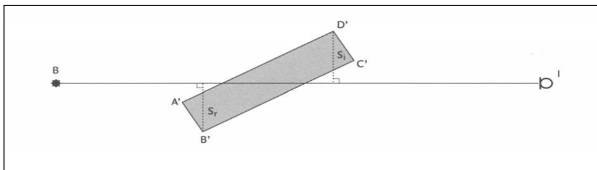
Figuur 3.4 Toelichting bij de bepaling van s_l en s_r bij een gebouw
