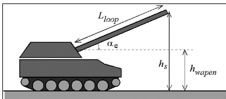
Figuur 4.1: Met de parameters h_{wapen} en L_{loop} kan de hoogte h_s van het bronpunt van de mondingsknaal worden berekend voor een gegeven elevatiehoek \alpha_e . In deze afbeelding valt het bronpunt samen met de vuurmond, maar in het algemeen kan het bronpunt op enige afstand van de vuurmond liggen. L_{loop} is dan langer dan de feitelijke lengte van de loop (zie § 4.5.1).
